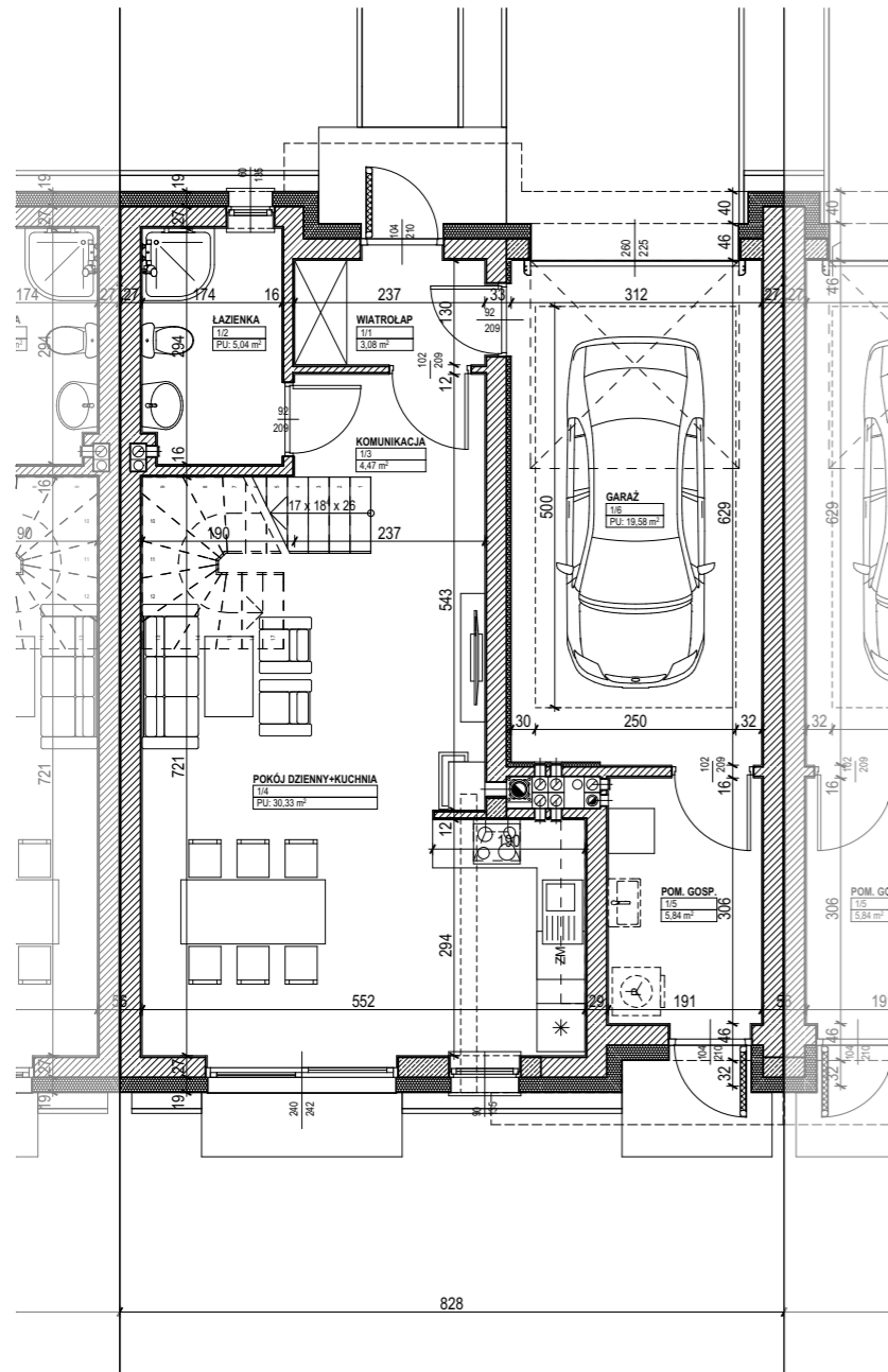
Parter MAJOLIKOWA 27R 1:100
